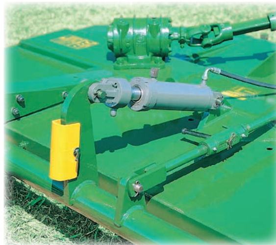
Regulador da altura de corte no cilindro. Varão estabilizador para nivelamento da roçadeira.
