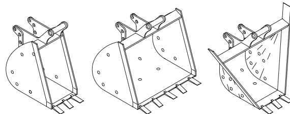
Caçambas de 12", 16", 18", 20" e 24"
